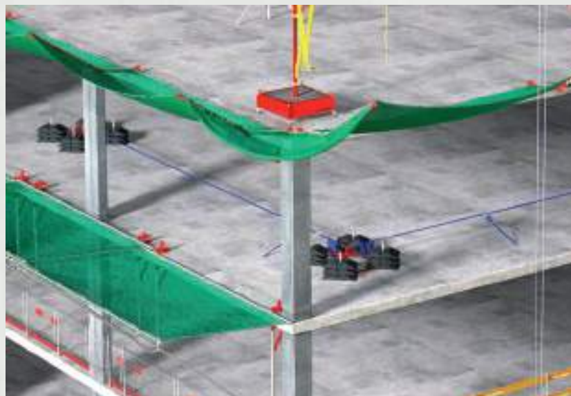
Linia życia podpięta do balastów bezwładnościowych „SPIDER”.
